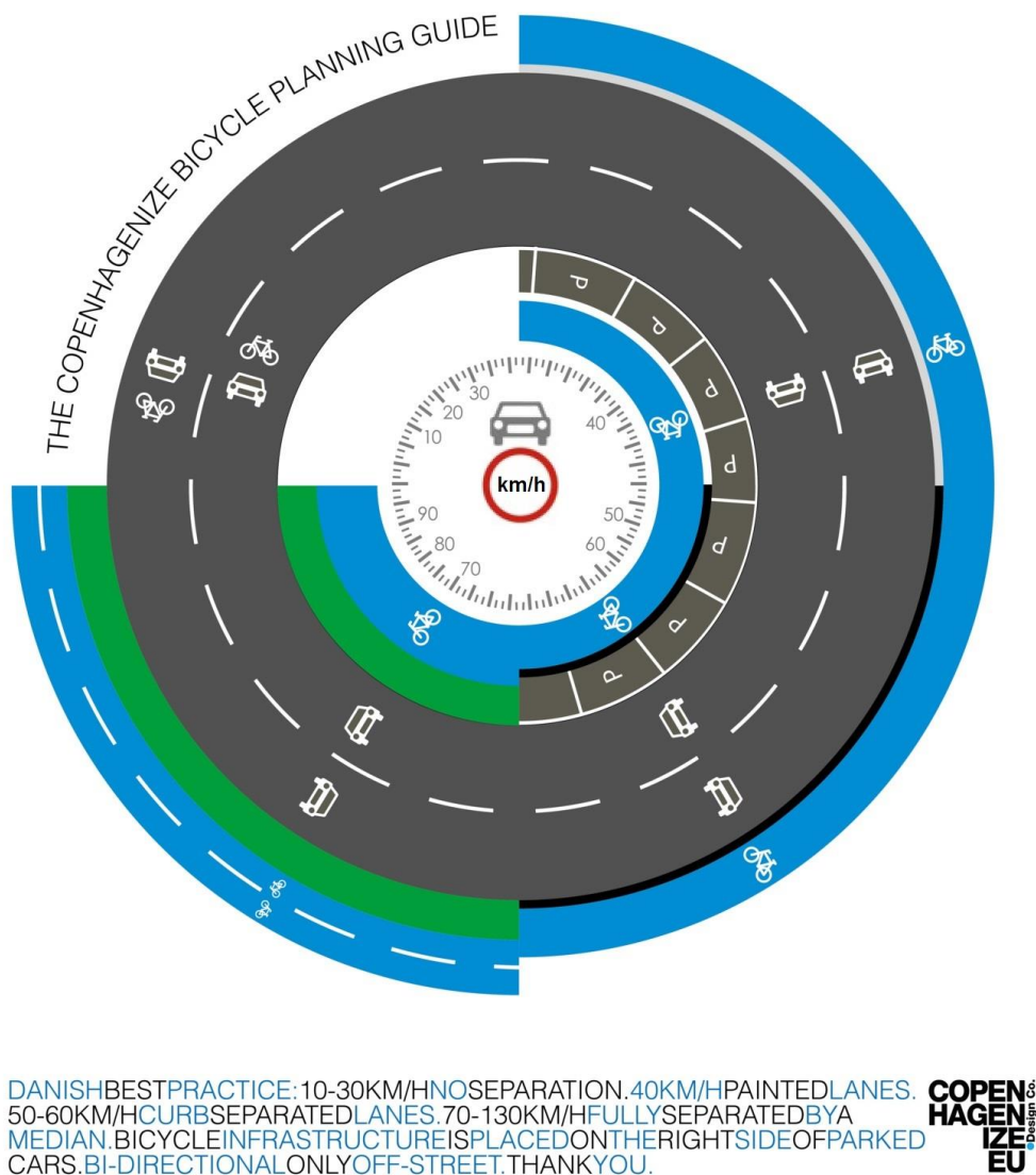
Fig. 8: Esquema de selecção do tipo de percurso ciclável.
