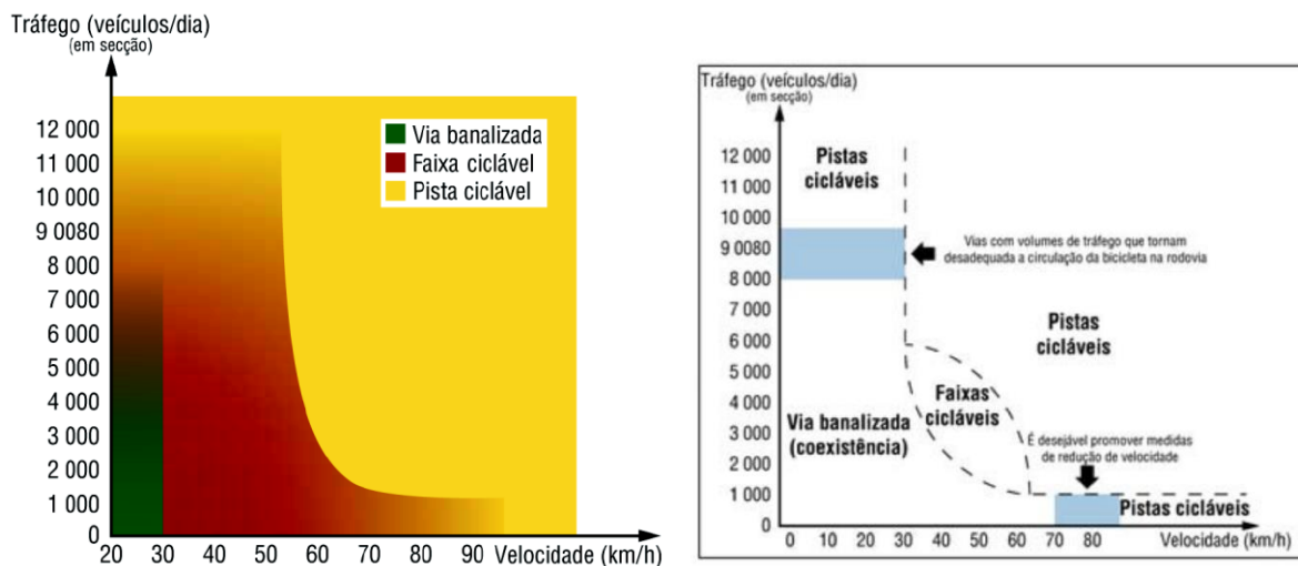
Fig. 7: Selecção do tipo de percurso ciclável em função da velocidade e volume de tráfego.
